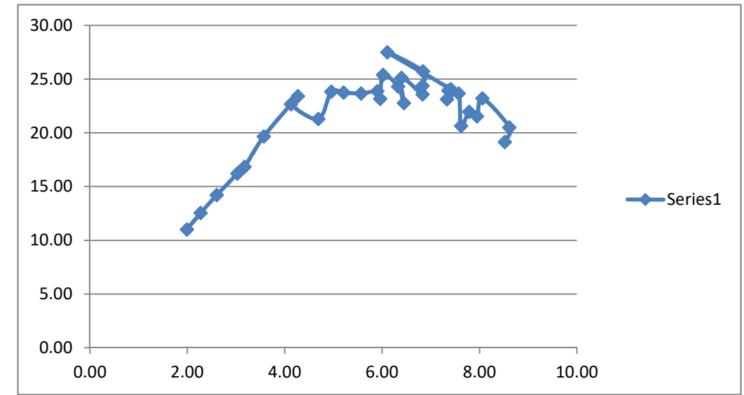
Mars over Jupiter 0.3 degrees away
